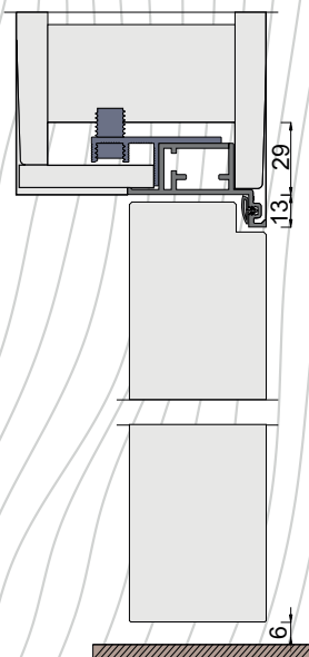
inward opening
